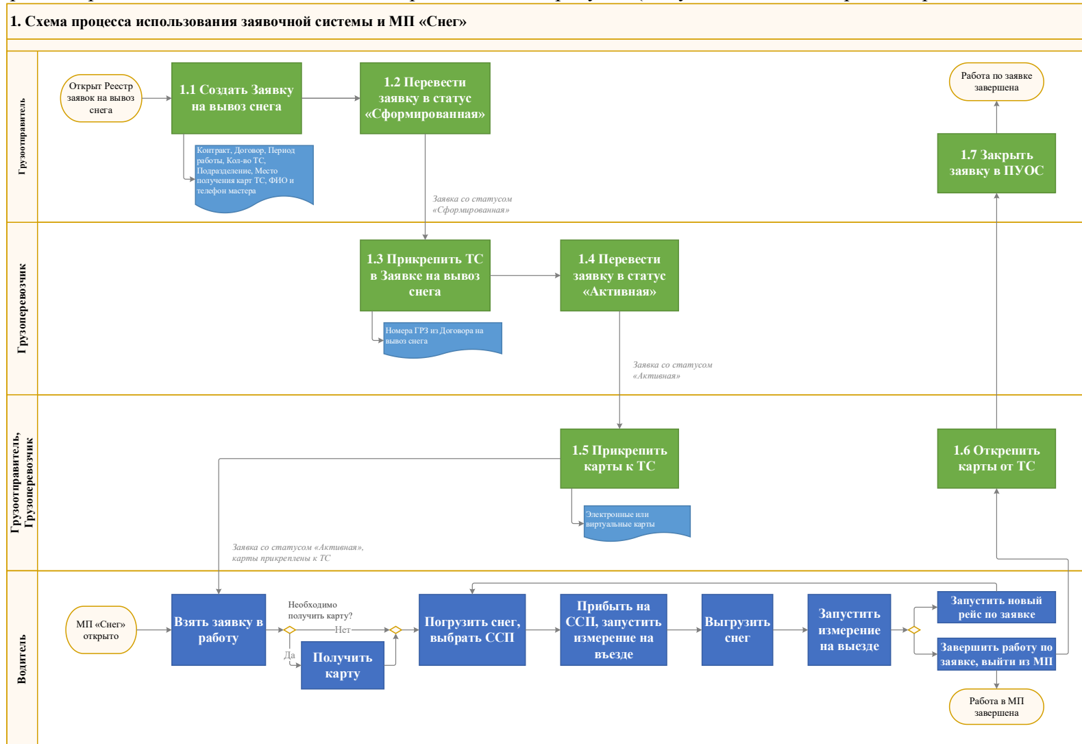
Рисунок 85 - Схема процесса работы с Заявкой на вывоз снега
