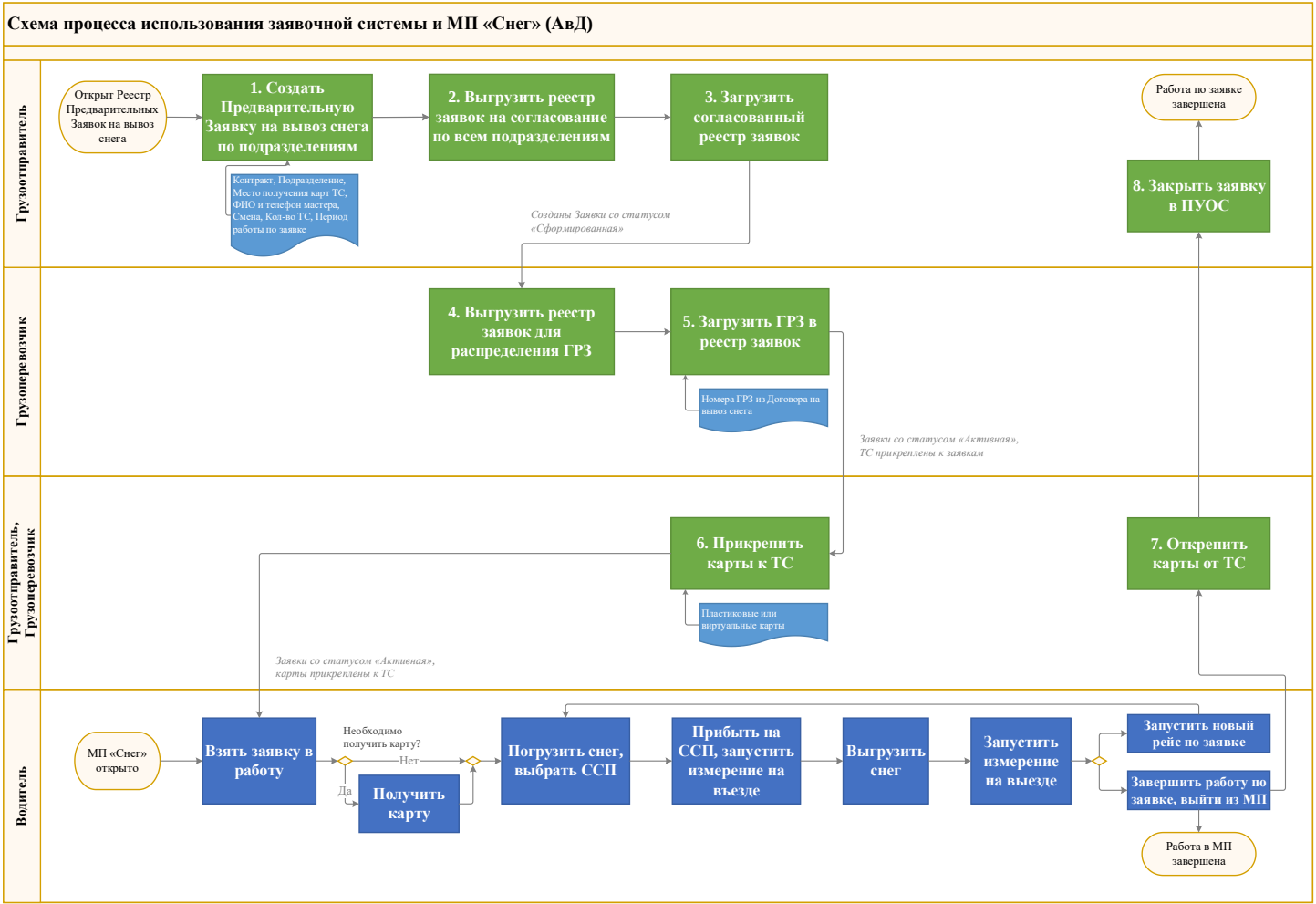
Рисунок 70 - Схема процесса работы с Заявкой на вывоз снега
