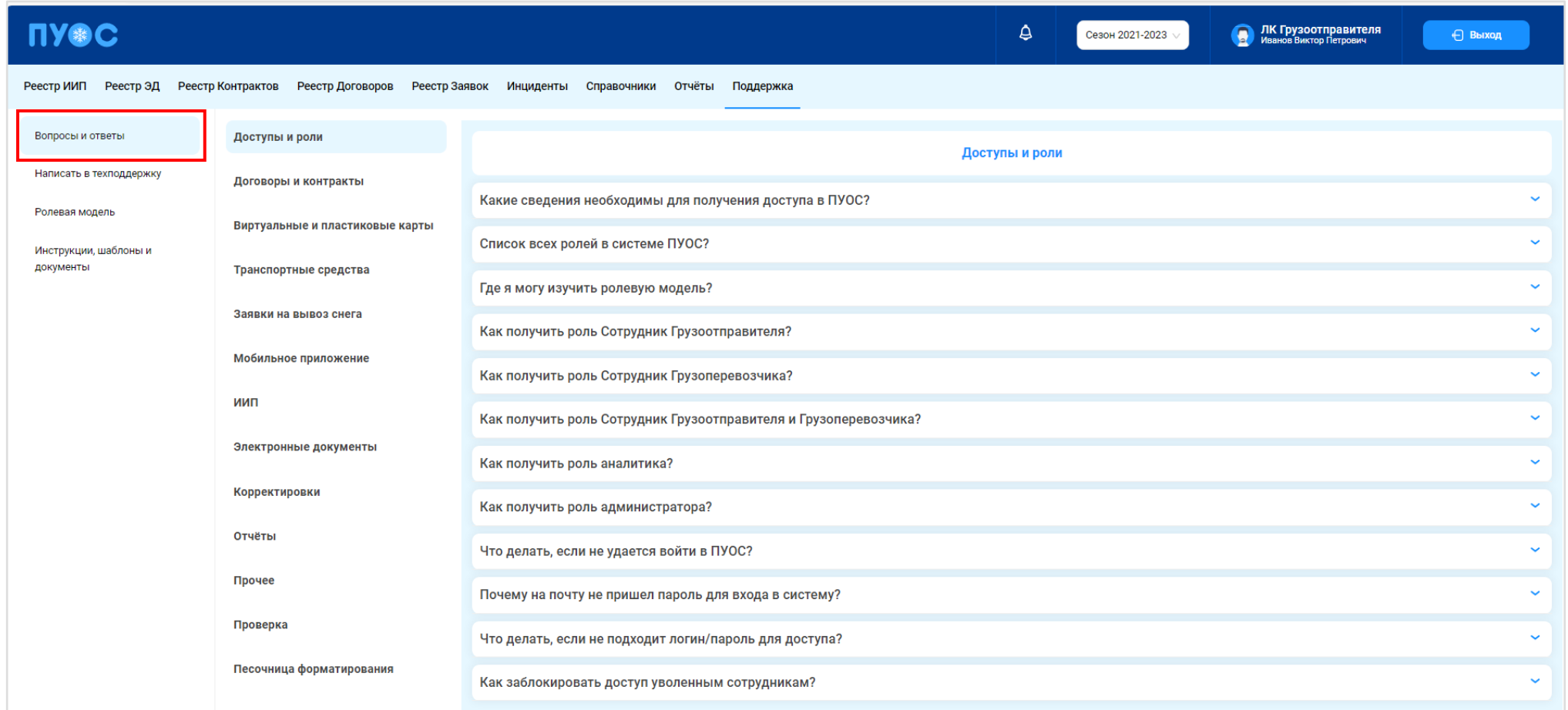
Рисунок 136 - Главная экранная форма подраздела «Вопросы и ответы»
